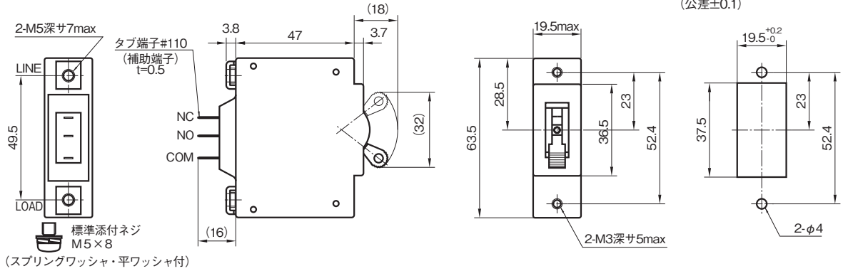
取付穴加工図 (公差±0.1)
