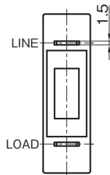
基板穴加工図 (公差±0.1)
