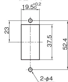
取付穴加工図 (公差±0.1)
