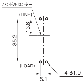
[回路形式 1・9]
