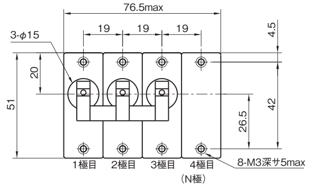
取付穴加工図 (公差:±0.1)
