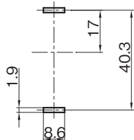
基板穴加工図 (公差±0.1)
