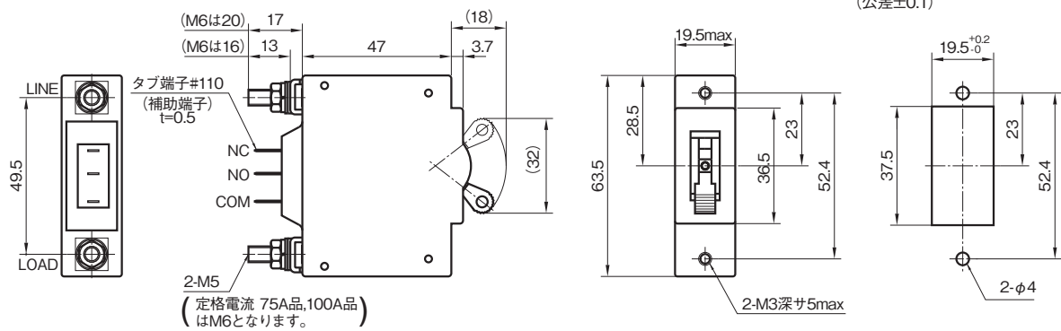
取付穴加工図 (公差±0.1)
