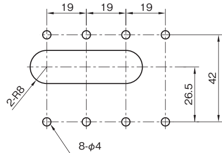
取付穴加工図 (公差:±0.1)
